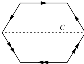
Figure 5: The jester’s hat
