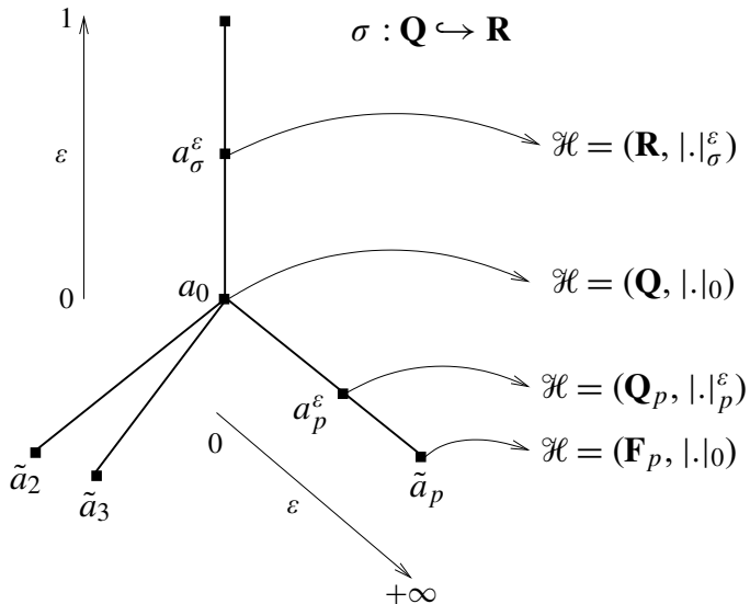
FIGURE 2. L'espace \mathcal{M}(\mathbf{Z}) .
